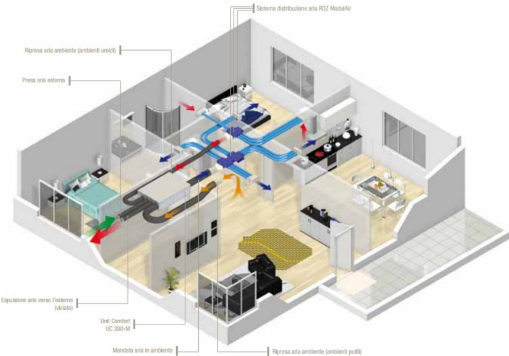
Impianto di riciclo dell'aria
